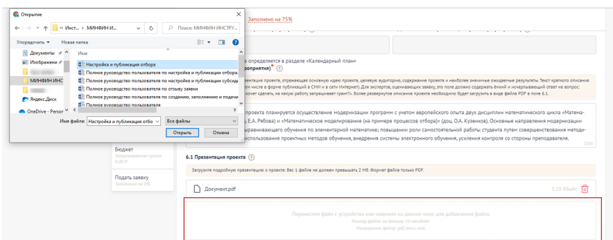
Рисунок 50. Диспетчер загрузки
