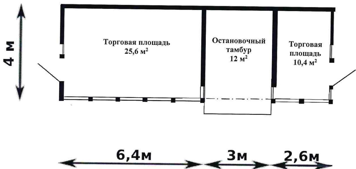
Вид сверху
