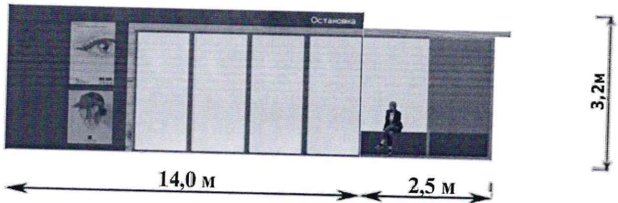
Главный фасад (длина) - Вариант № 2
